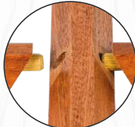
Petits bois extérieurs assemblés par tourillons et montés au cadrage de l'ouvrant.
