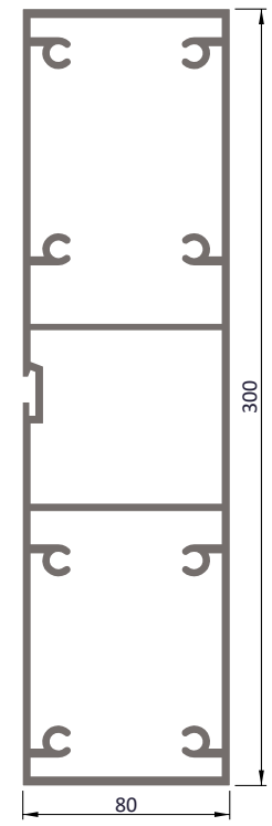
Profil poutre Plus • Beam Plus profile
