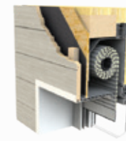
Demi-linteau ossature bois
