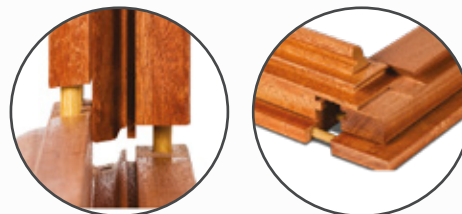
Assemblage des dormants et ouvrants en contre-profil et tourillons collés.
